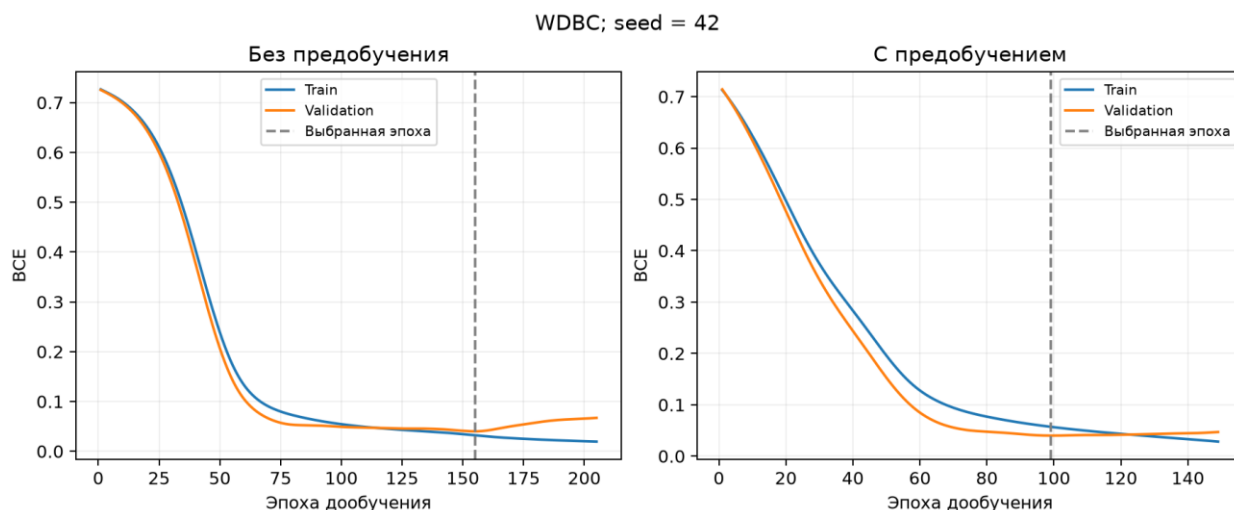
Рисунок 4 — Supervised-дообучение WDBC при seed 42
