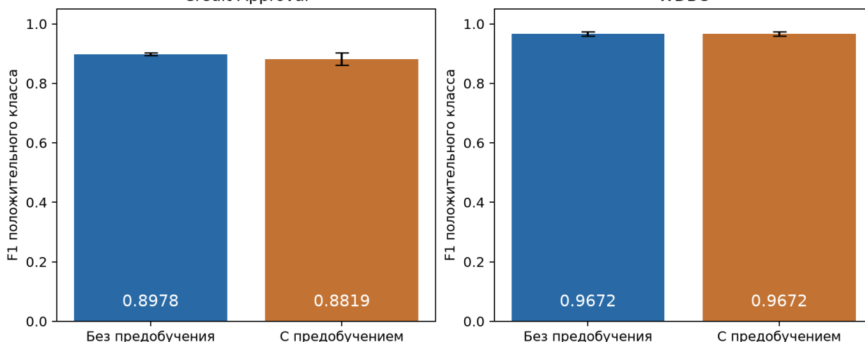
Рисунок 6 — Средний F1 и его разброс по трём инициализациям
