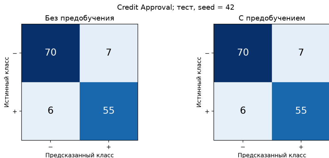
Рисунок 3 — Матрицы ошибок Credit Approval на тесте при seed 42
