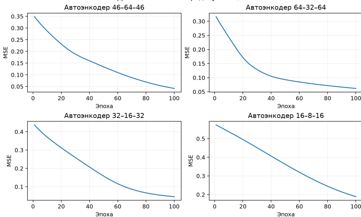
Рисунок 1 — Обучение четырёх автоэнкодеров Credit Approval
